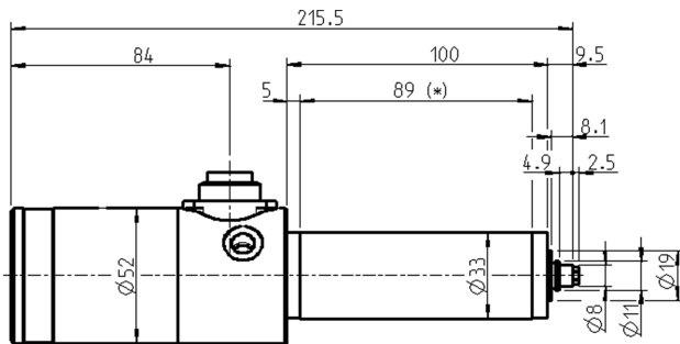
Abmessungen
