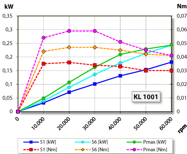
Leistungsdiagramm
